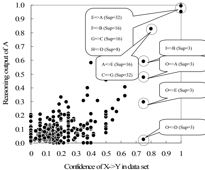
圖4：數值例題的ARNN的推論輸出值與資料中的信賴度之關係(隱藏單元數=2)
