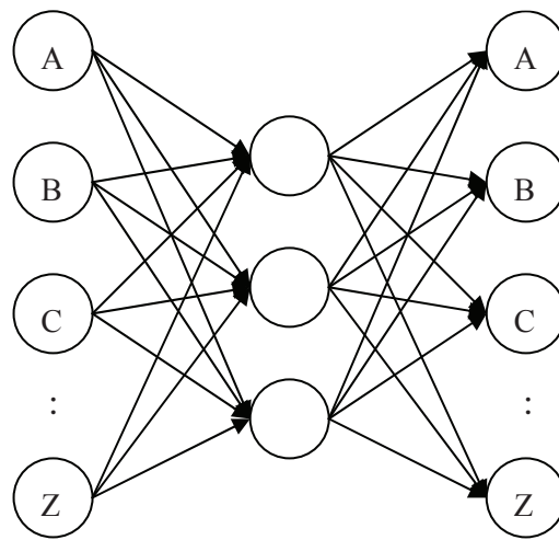
圖1：ARNN的架構
