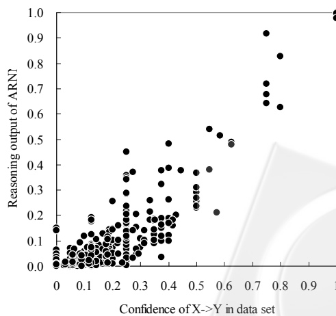
圖2：數值例題的ARNN的推論輸出值與資料中的信賴度之關係(隱藏單元數=8)
